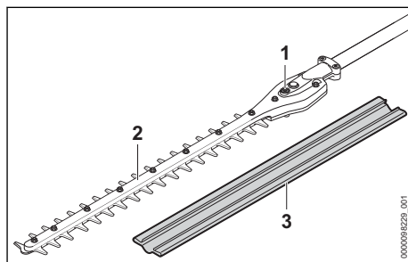
Niet-verstelbaar mes
