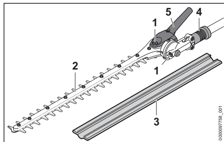
Verstellbares Schneidmesser
