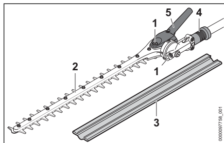
Verstelbare messen
