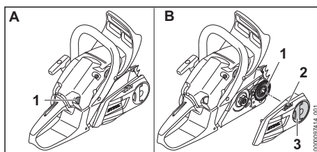
Kraftstoffhandpumpe (A)
