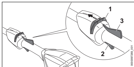
Pestillo de retención (1), gatillo (2) y palanca Ergo (3)
